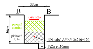
B - chodník NN kabel Rýha 35/50cm
