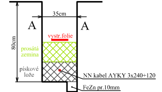
A - volný terén NN kabel Rýha 35/80cm
