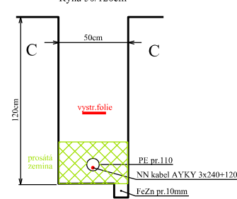
C - překop NN kabel Rýha 50/120cm
